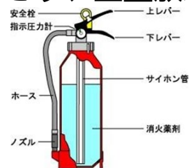
【蓄圧式消火器】
