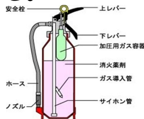
【加圧式消火器】
